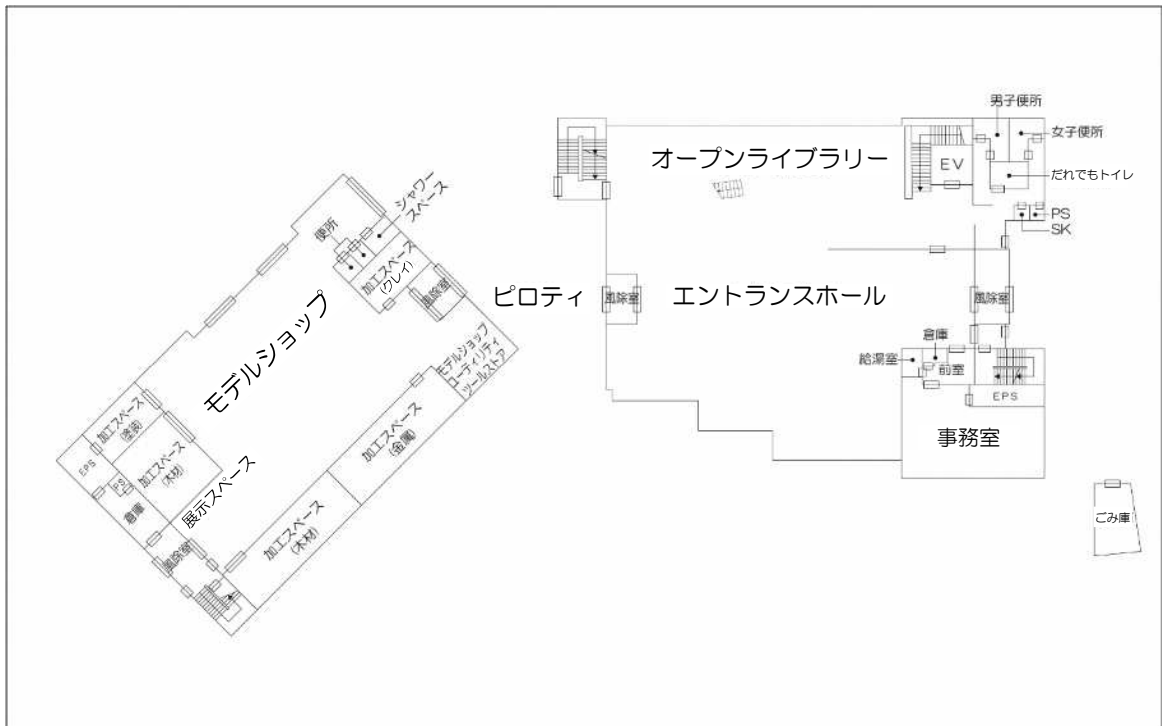
1 階 平 面 図
