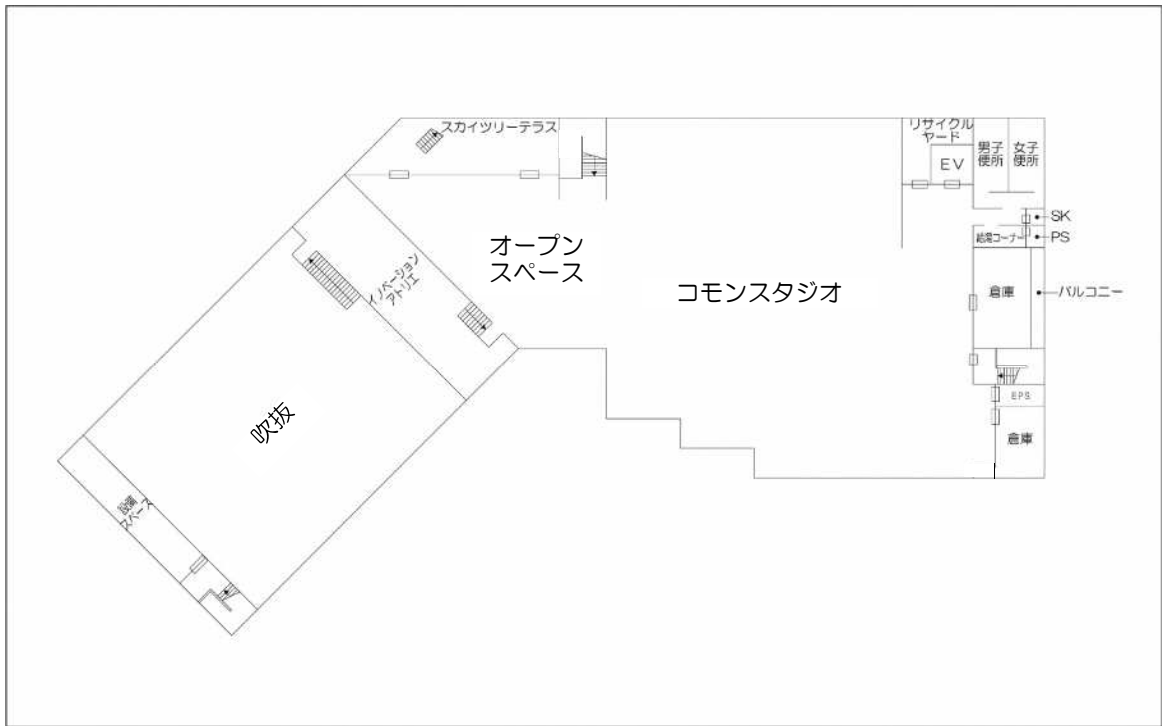
5階平面図
