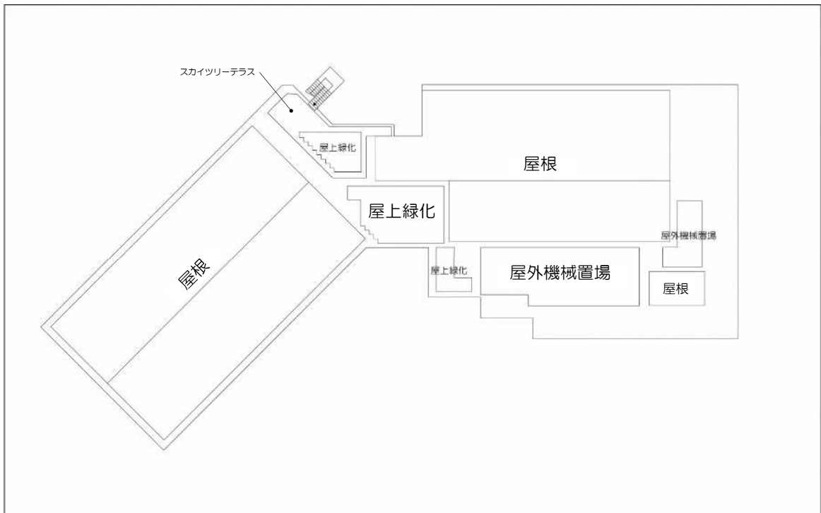
屋上平面図
