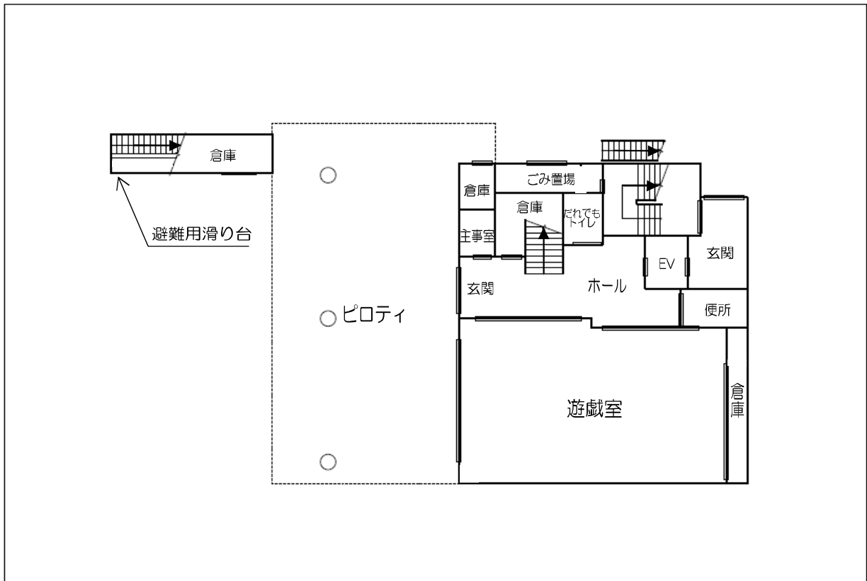
1階平面図
