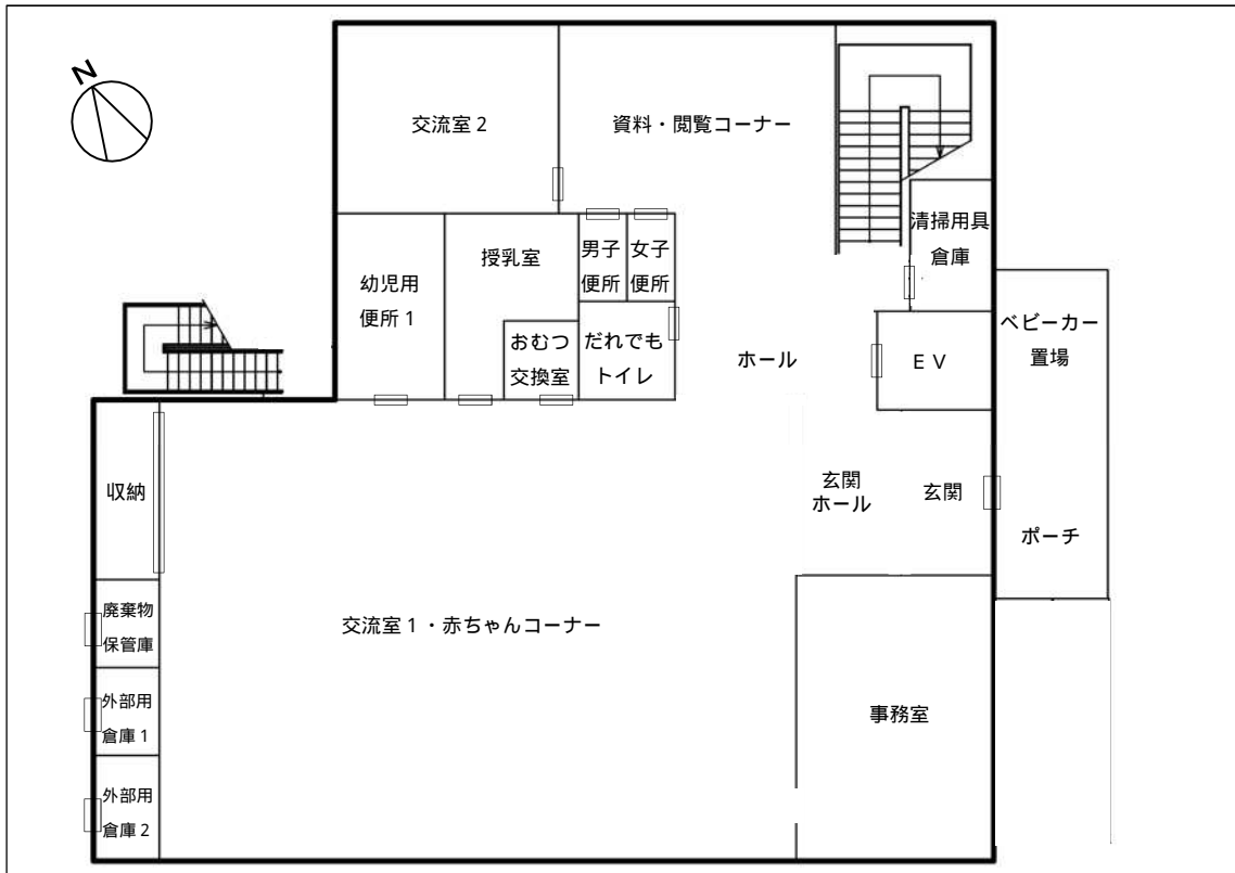
1階平面図
