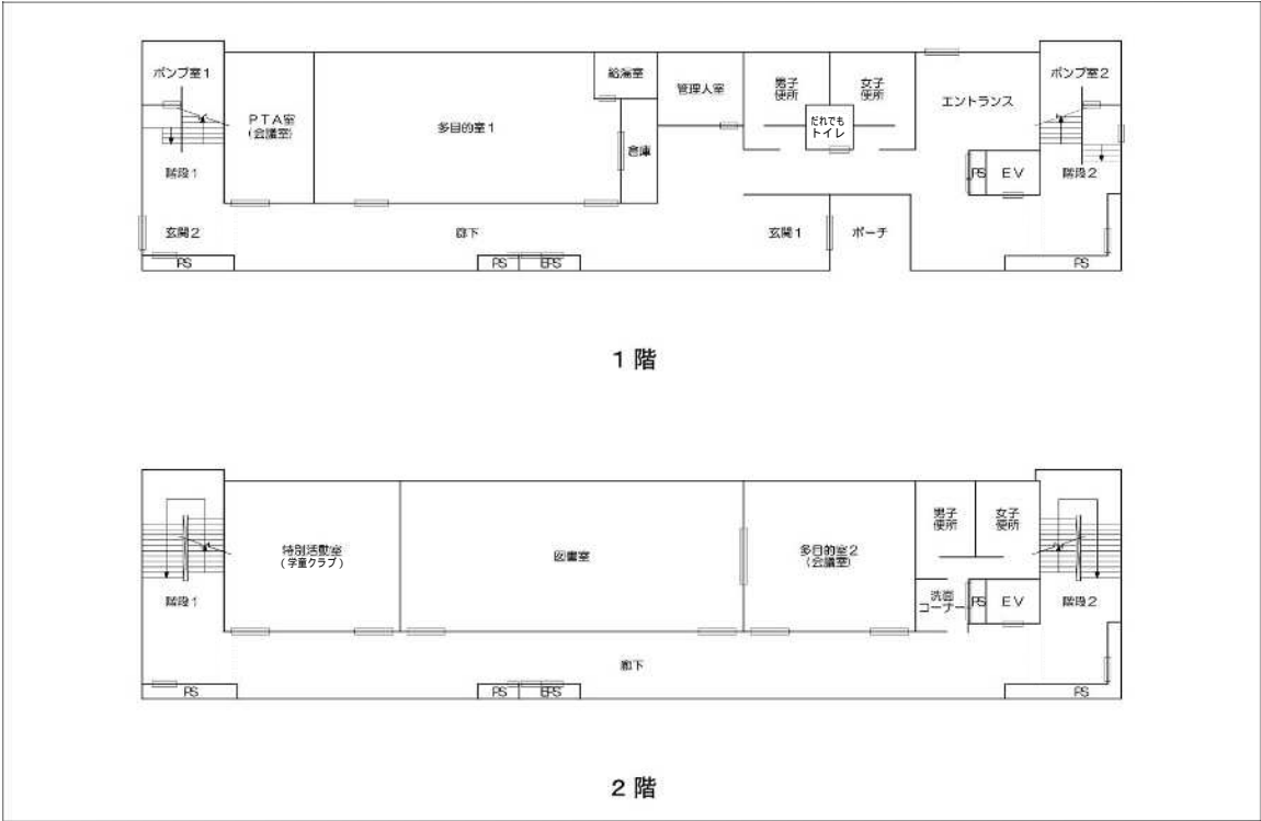
1階・2階平面図
