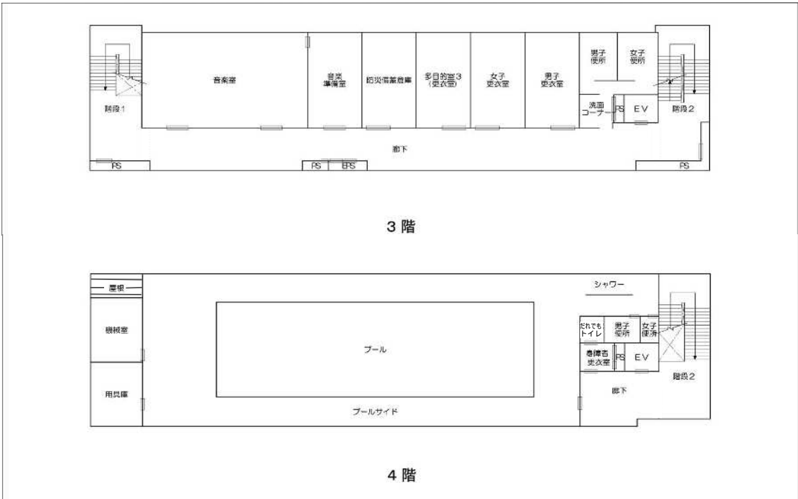
3階・4階平面図
