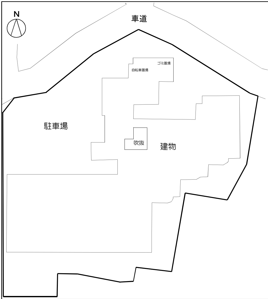
配置図
