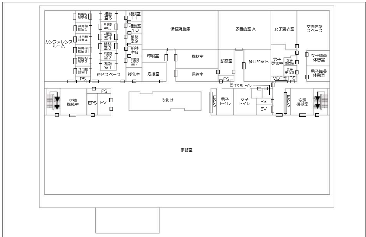
2 階 平 面 図
