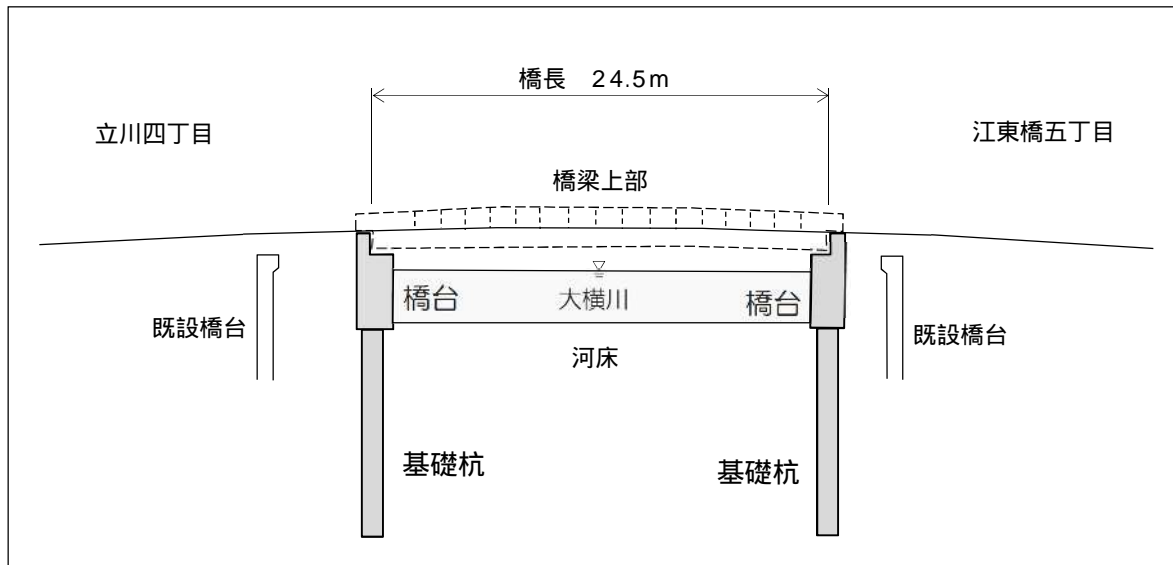
側面図
