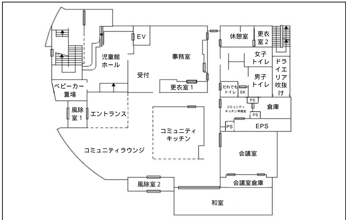
1 階 平 面 図
