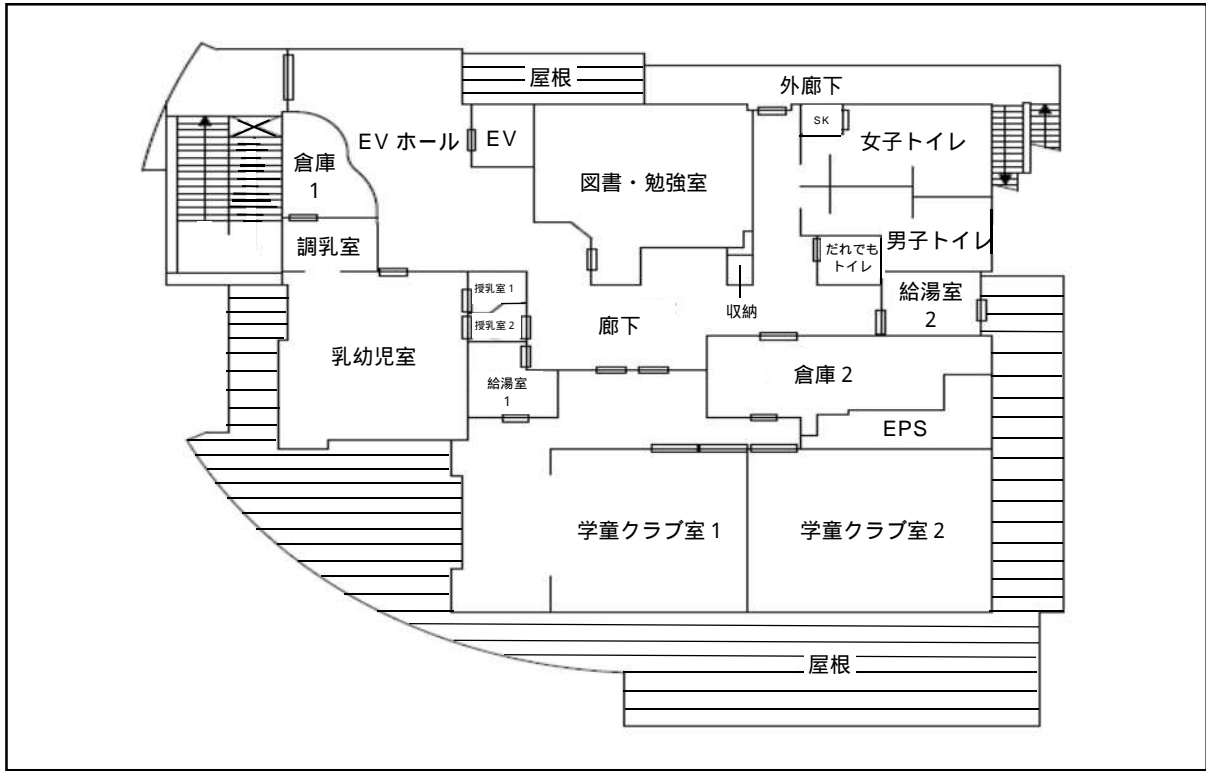
3 階 平 面 図
