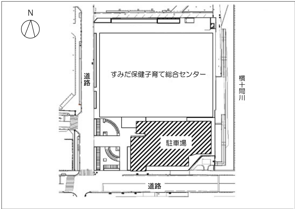
配置図
