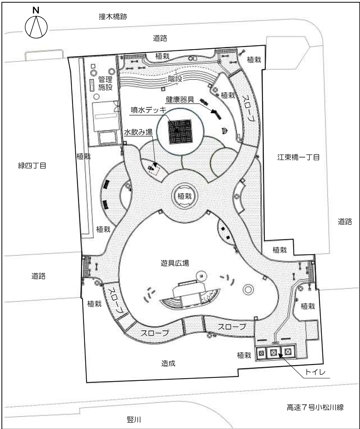
平面図
