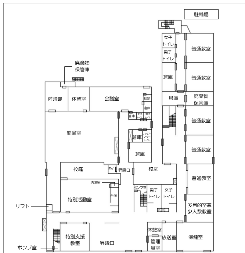
1 階 平 面 図
