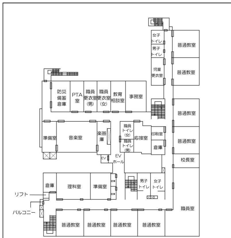
2 階 平 面 図
