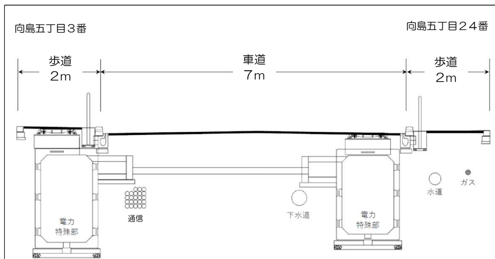
A-A' 断面図
