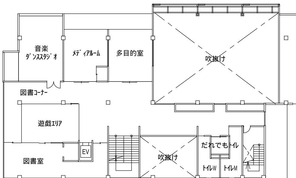
3 階平面図
