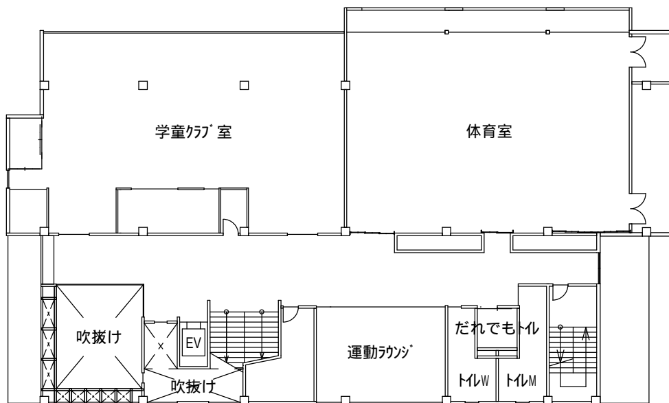
2 階平面図
