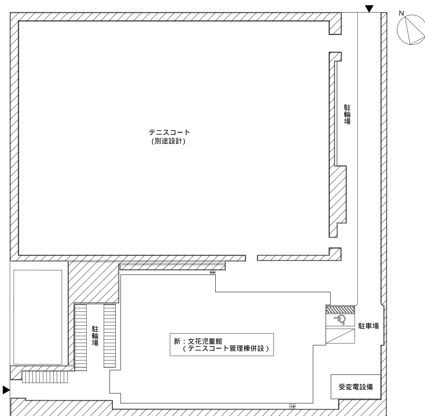
配置図
