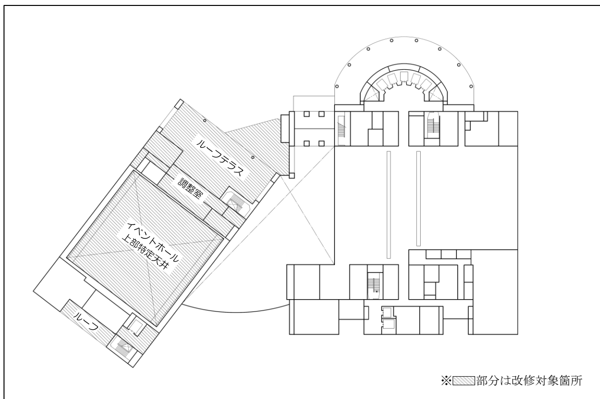
3 階 平 面 図
