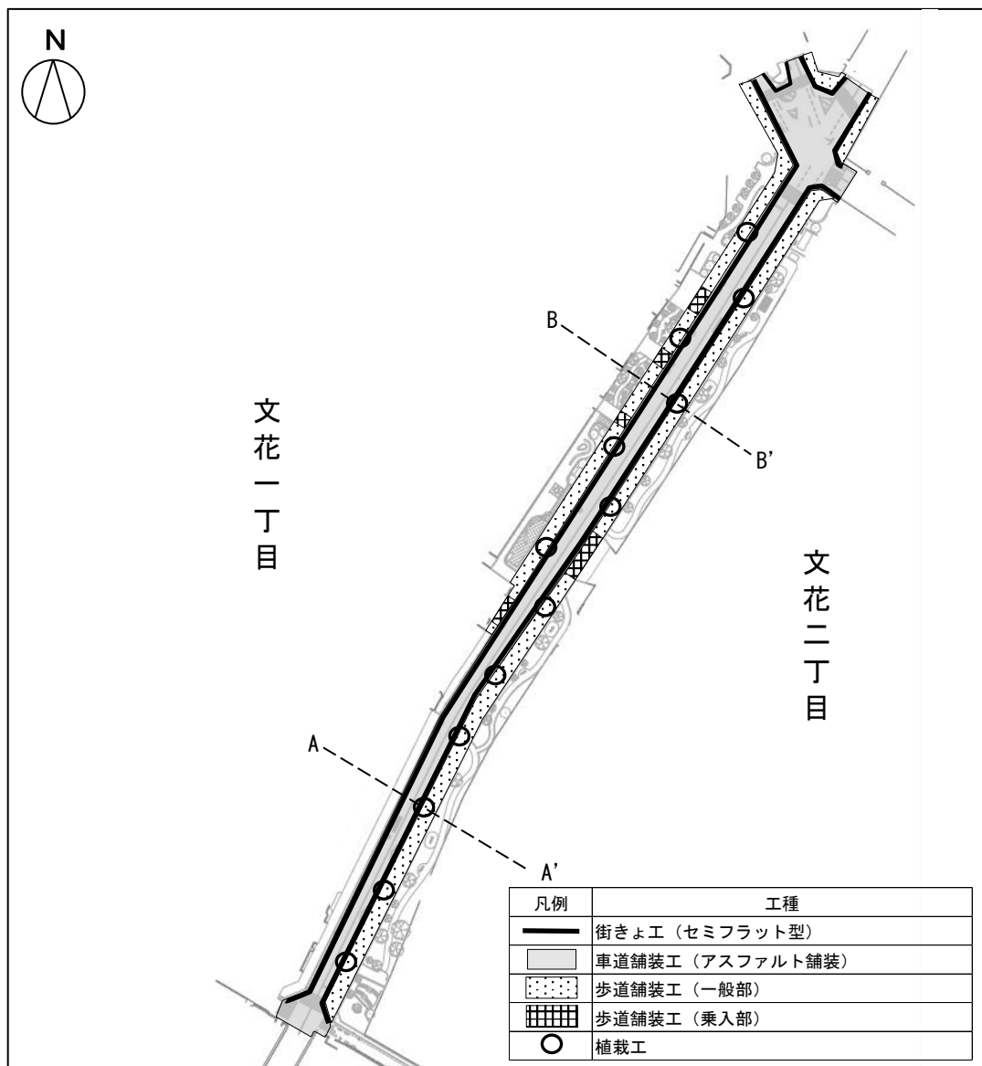
平面図
