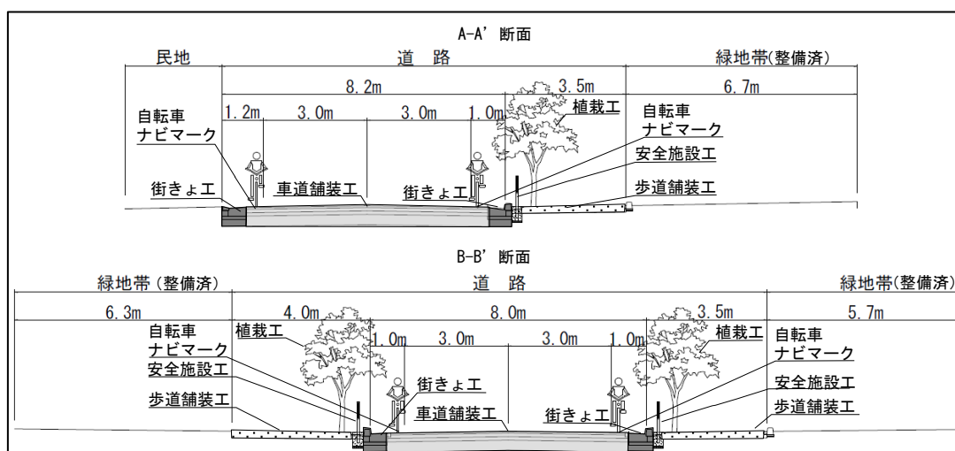
断面図
