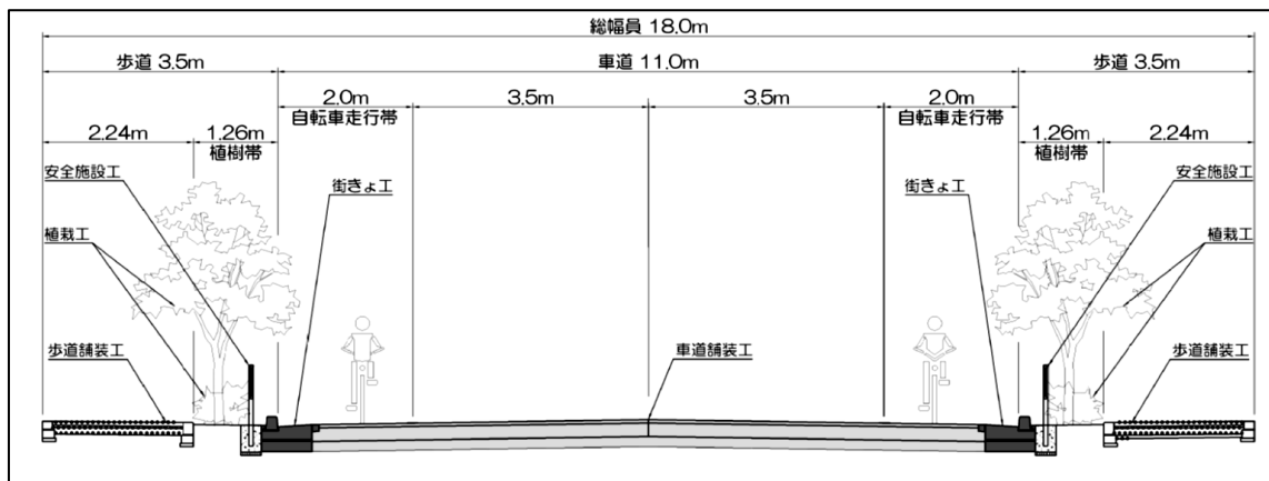
断面図
