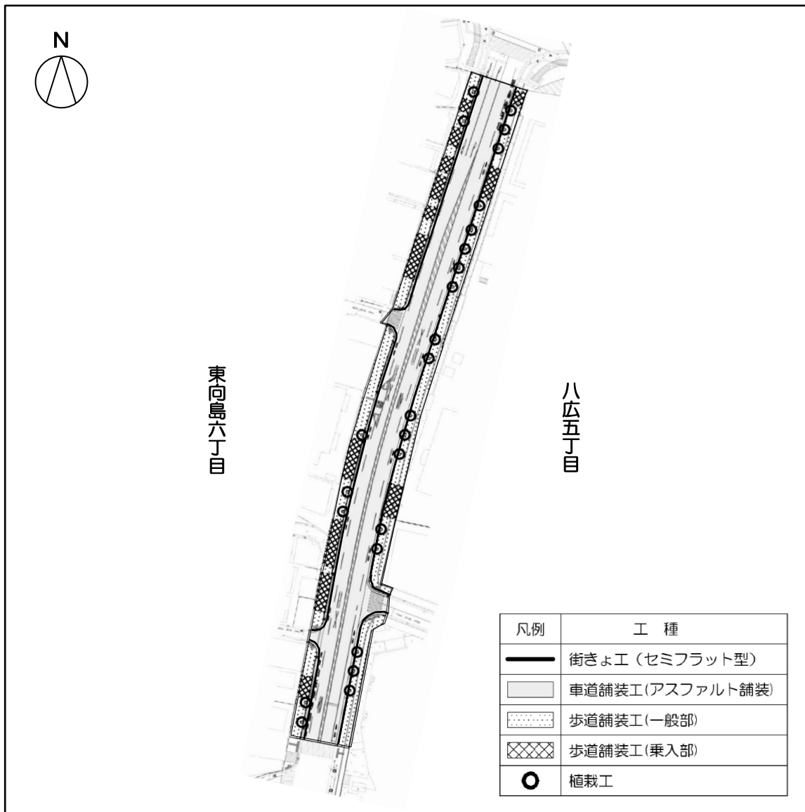
平面図
