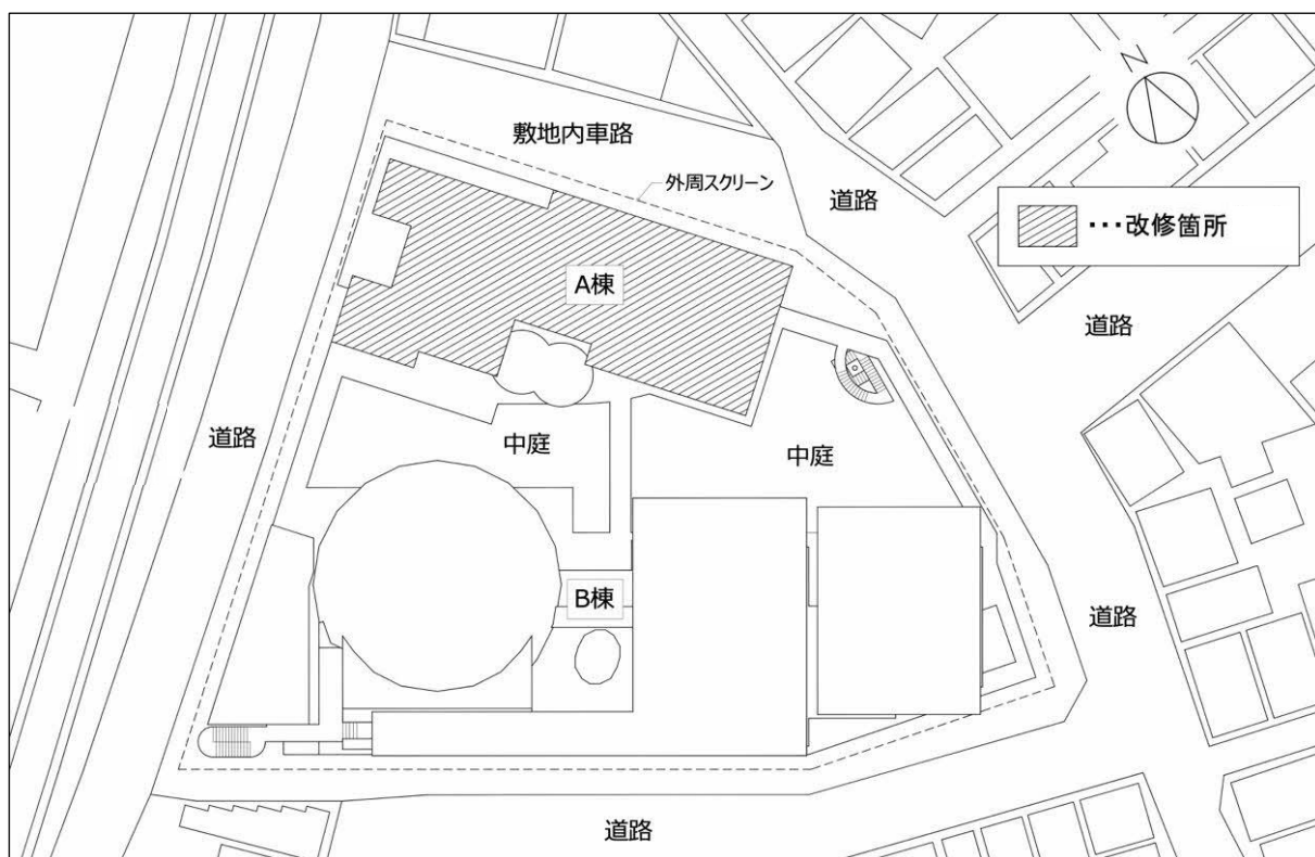
配 置 図
