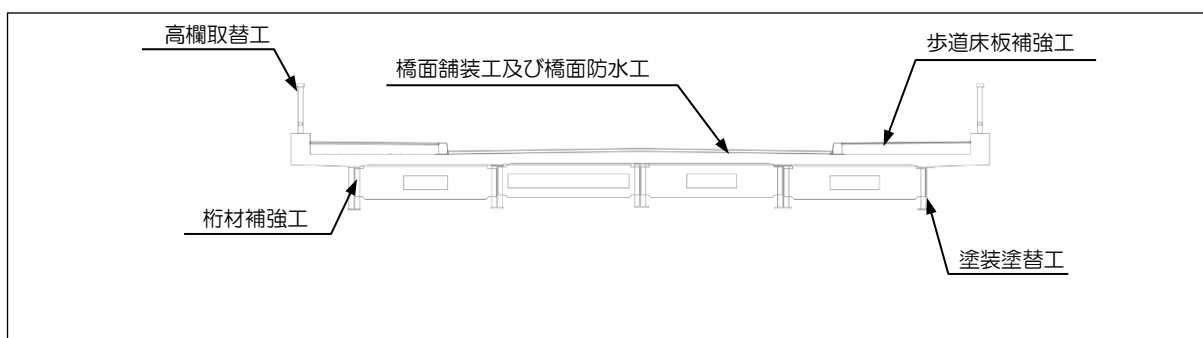
B - B'断 面 図
