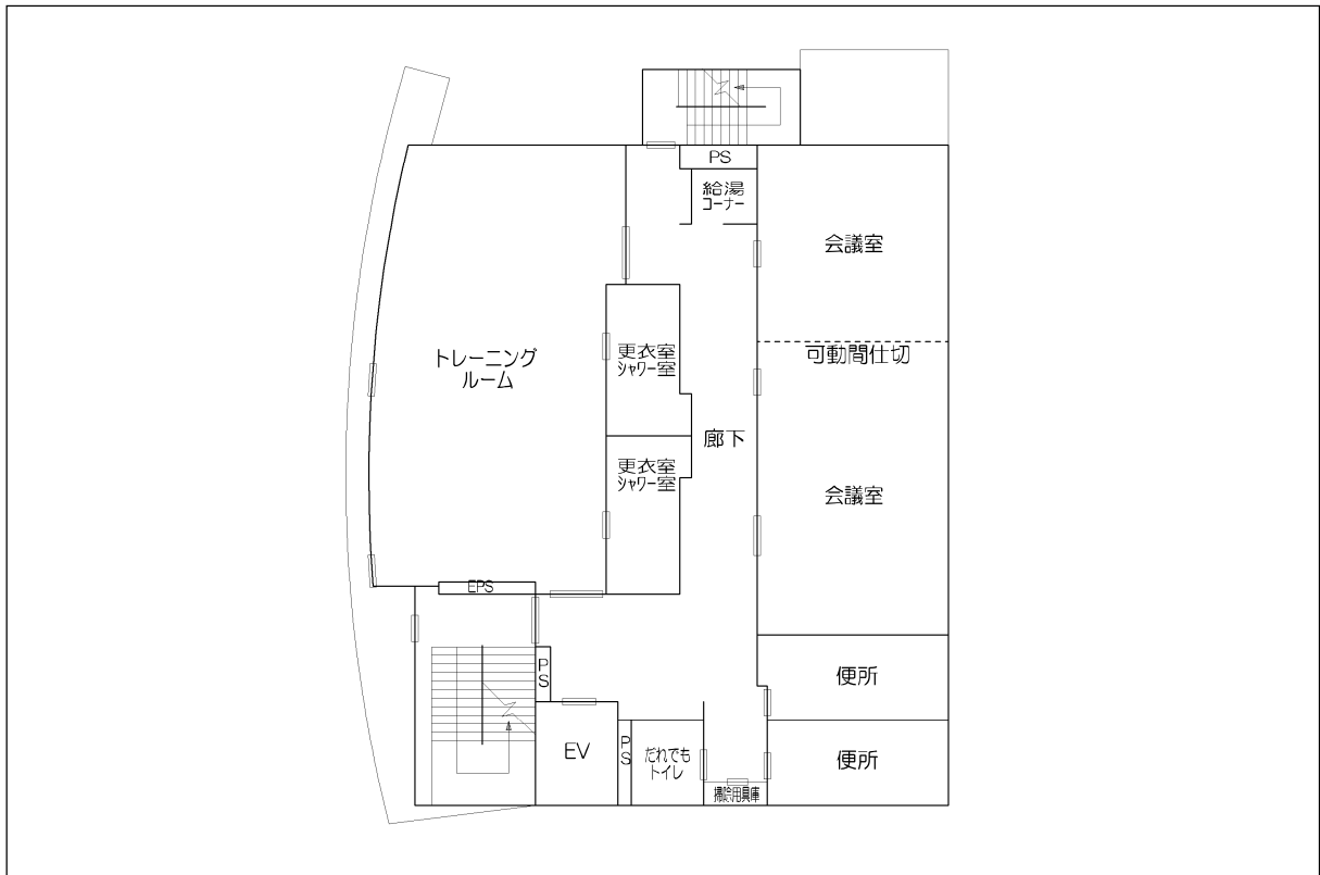
3 階 平 面 図
