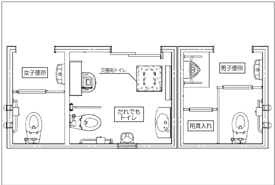
平 面 図
