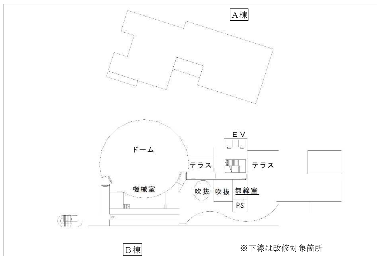
5 階 平 面 図
