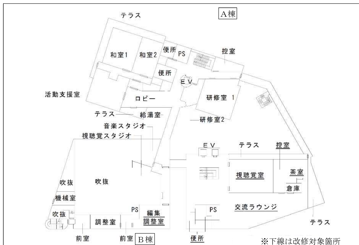
3 階 平 面 図
