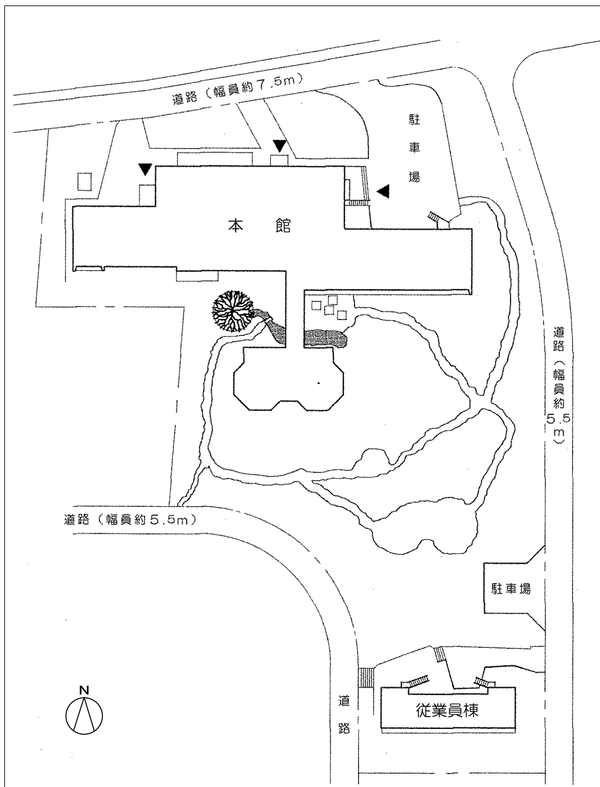
配 置 図
