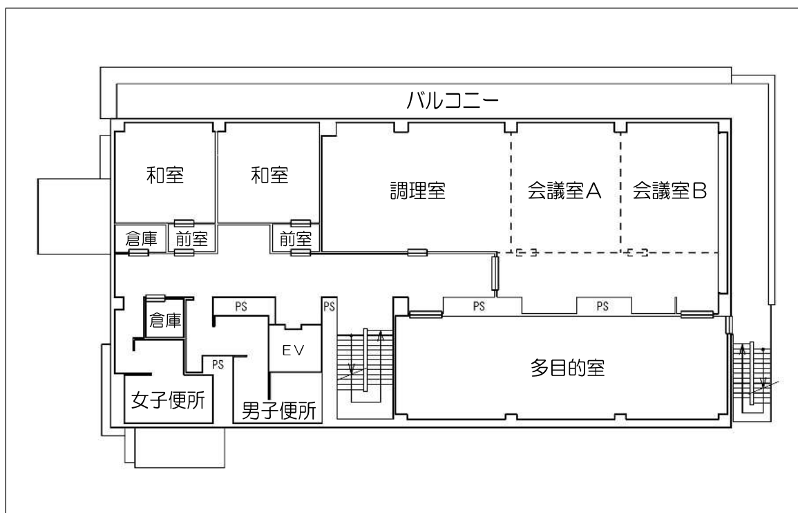
2 階 平 面 図（セミナーハウス）
