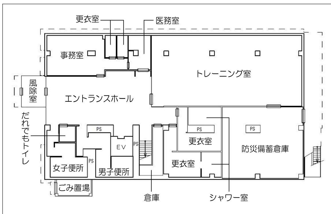
1 階 平 面 図（セミナーハウス）
