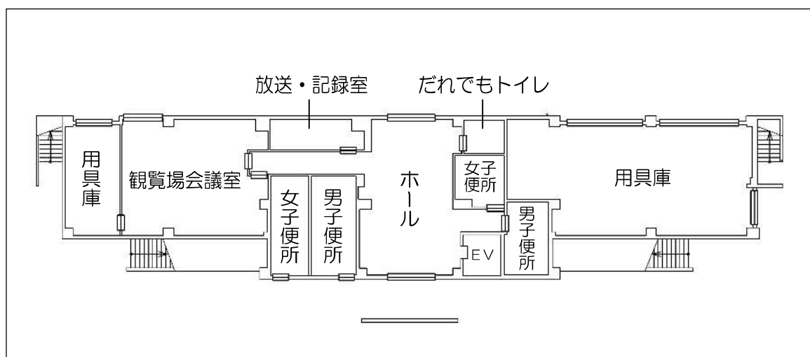
1 階 平 面 図（観覧場）
