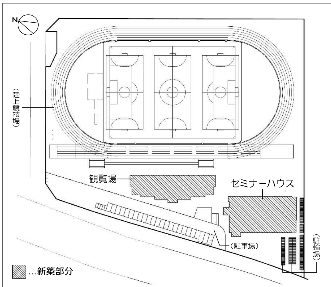
配 置 図
