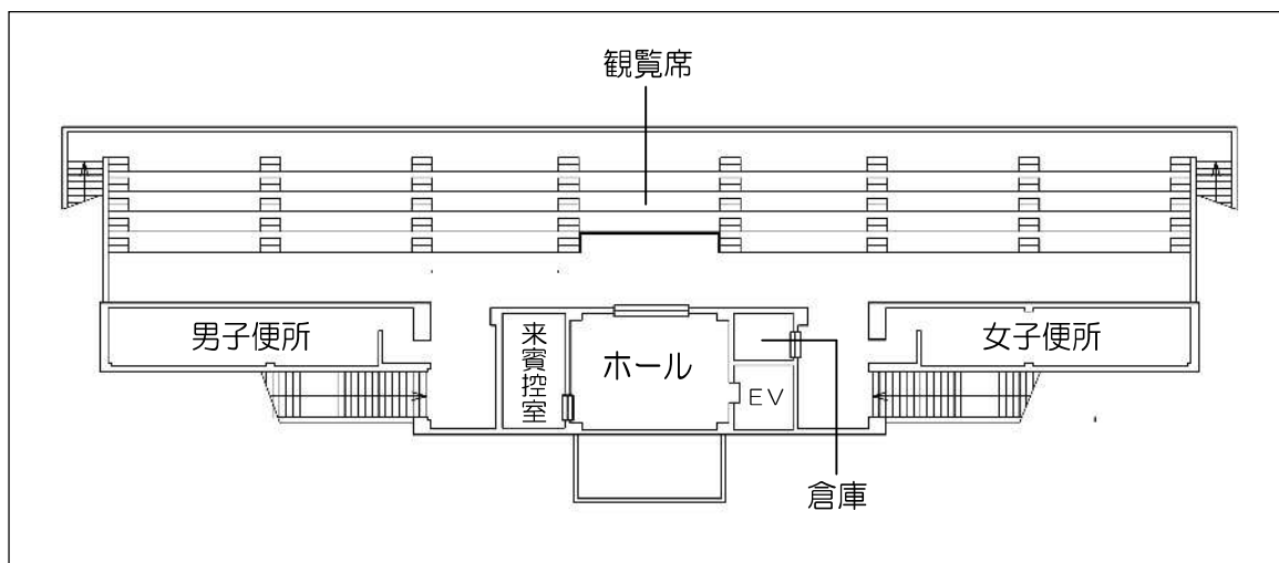
2 階 平 面 図（観覧場）
