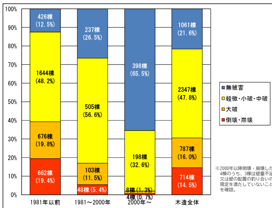
図 1-4-5 建築年代別の倒壊・崩壊の割合(能登半島地震)
