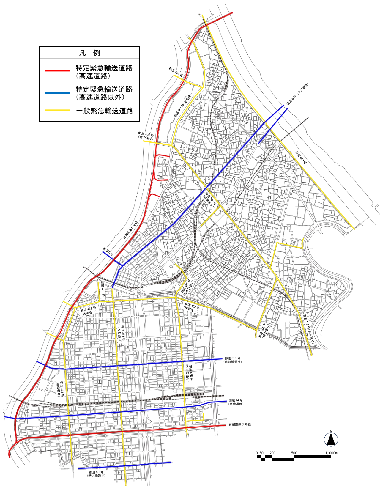
図 1-5-1 緊急輸送道路指定図 (令和 8 年 3 月末時点)
