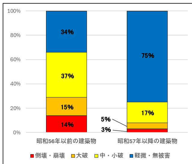
図 1-4-2 阪神・淡路大震災における昭和 56 年以前と昭和 57 年以降に建築された建築物の被害状況 出典：平成 7 年 阪神・淡路大震災建築震災調査委員会 中間報告
