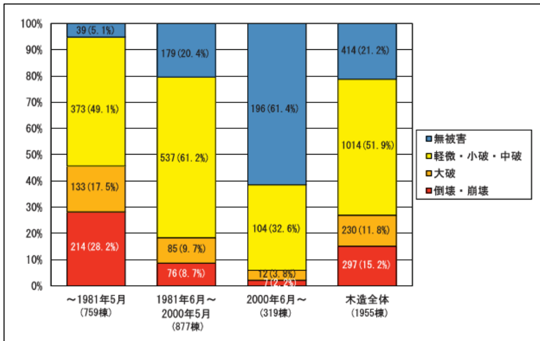
図 1-4-3 木造建築物の建築時期別の被害状況（益城町中心部における悉皆調査）
