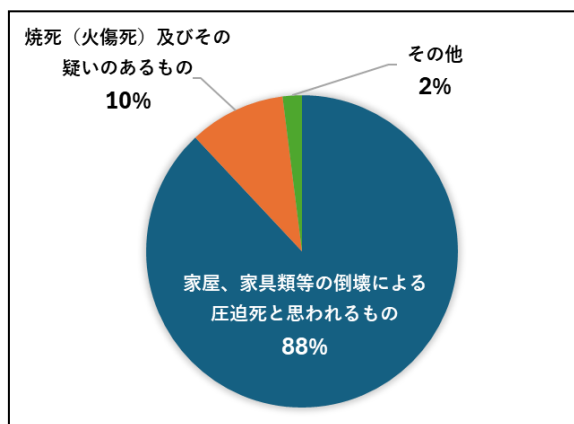
図 1-4-1 阪神・淡路大震災における死因 出典：平成 7 年 警察白書
