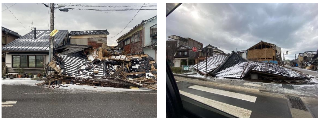
図 1-4-6 能登半島地震被害状況写真(区派遣職員撮影)
