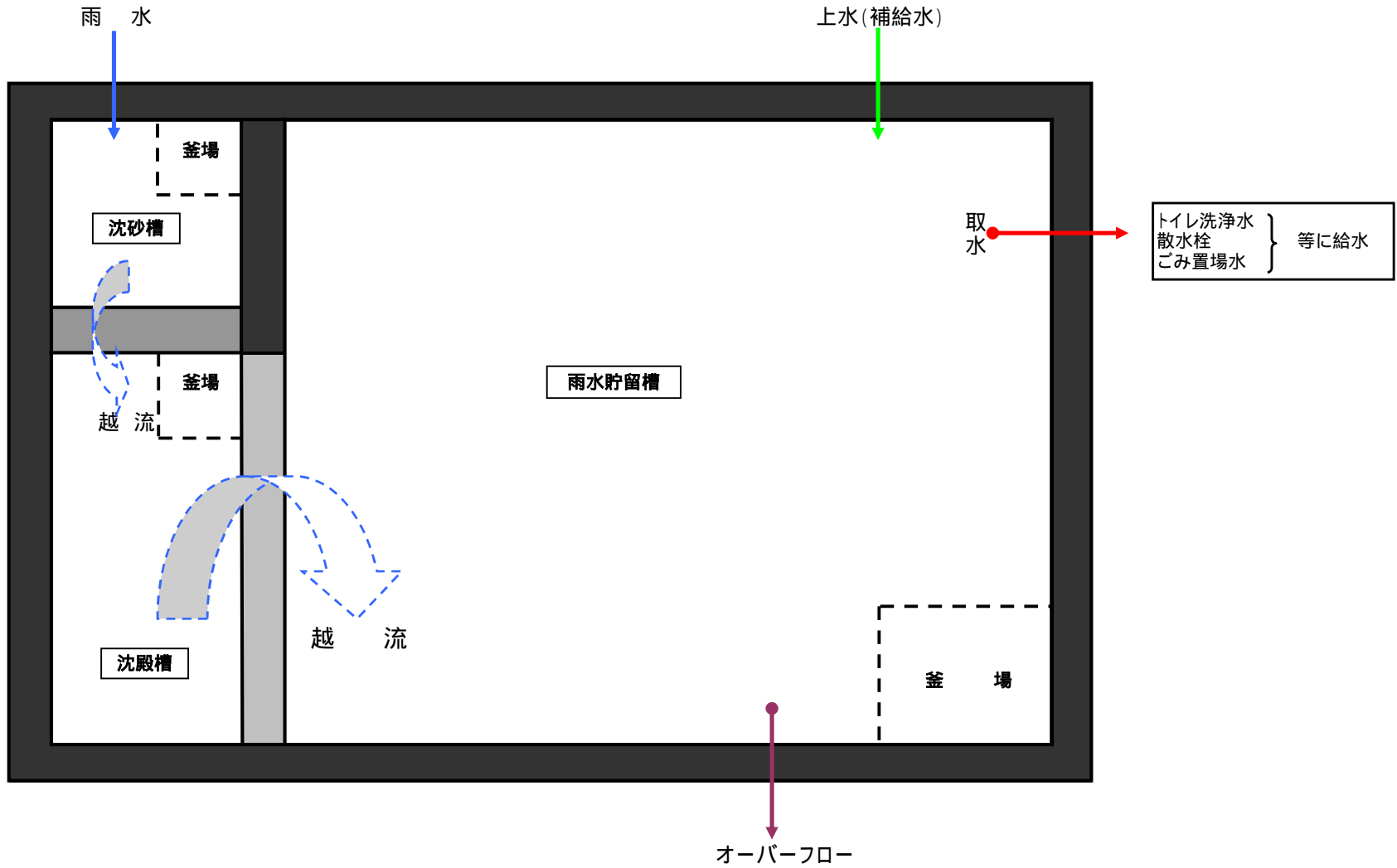
【雨水貯留槽平面図】
