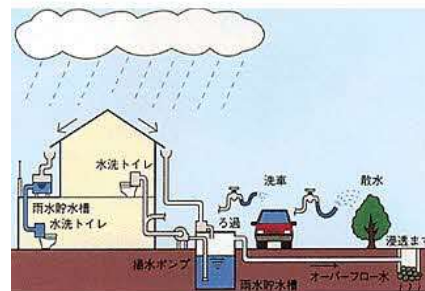
雨水貯留イメージ
