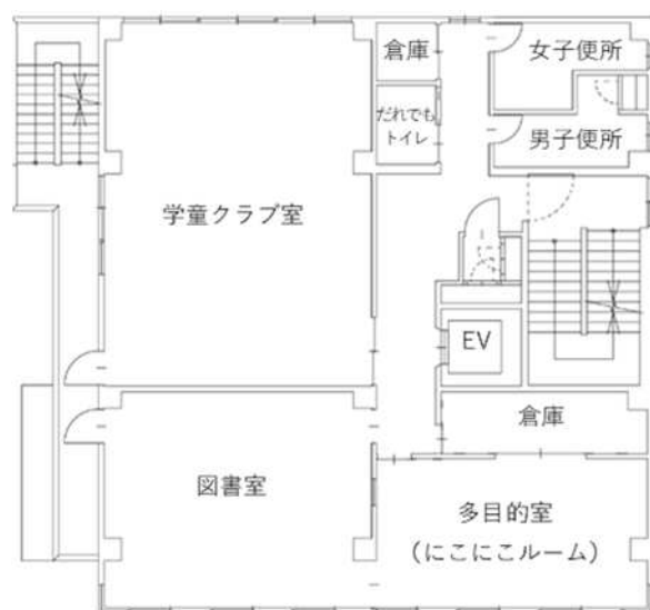
2 階平面図
