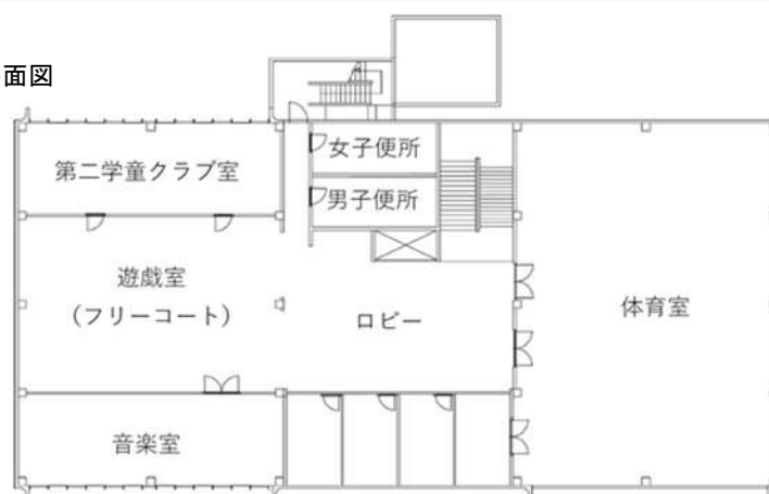
3 階平面図
