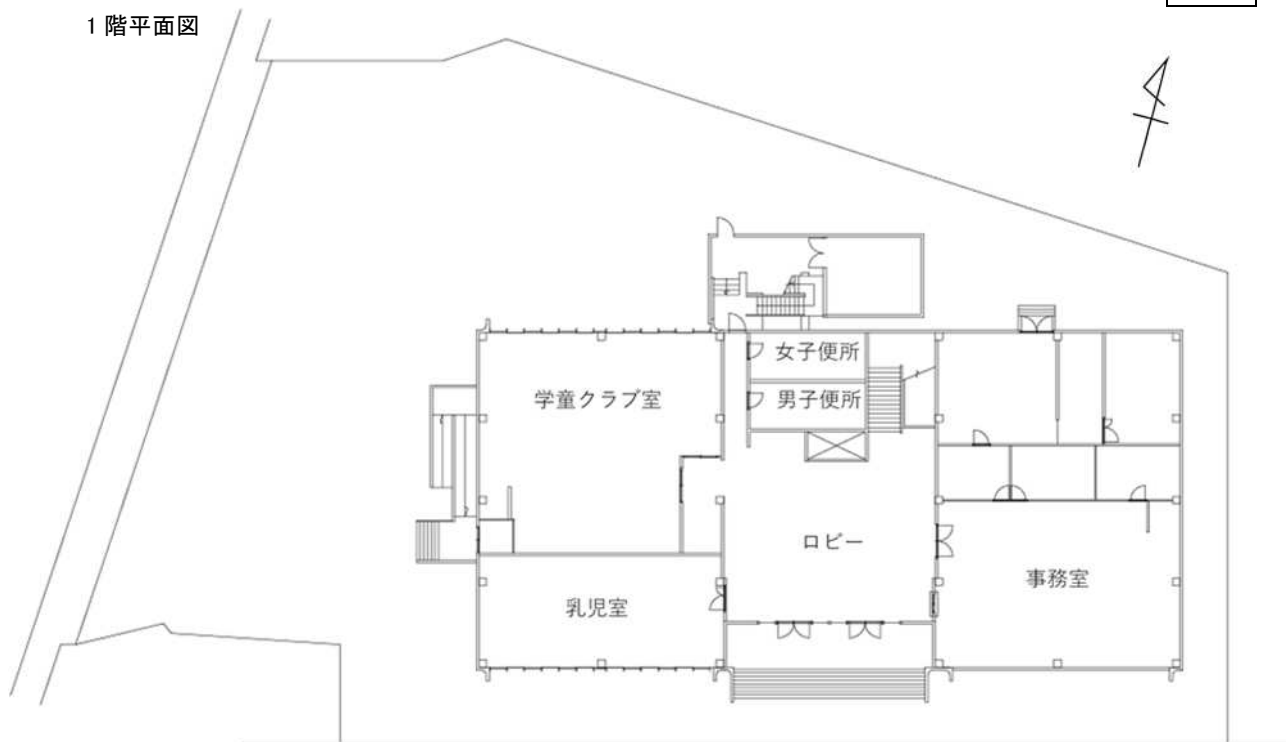
2 階平面図
