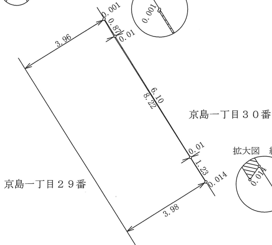
拡大図 縮尺1/1
