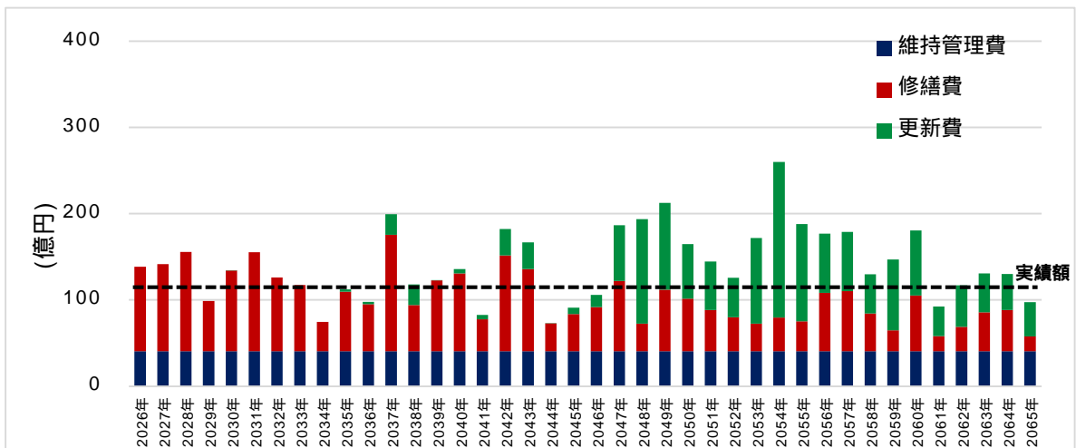
図3-4-7 目標使用年数をすべて80年と仮定した場合の試算結果グラフ
