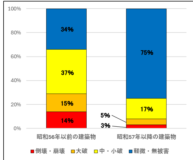
図 1-4-2 阪神・淡路大震災における昭和 56 年以前と昭和 57 年以降に建築された建築物の被害状況 出典：平成 7 年 阪神・淡路大震災建築震災調査委員会 中間報告
