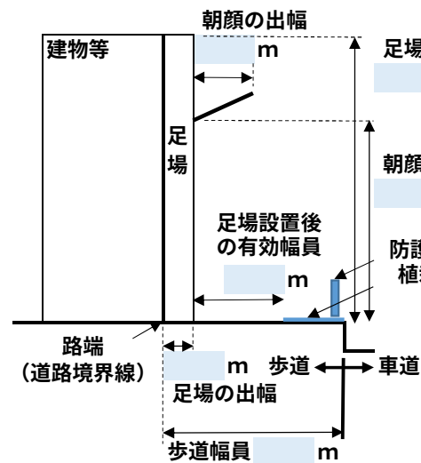
断面図(側面図)
