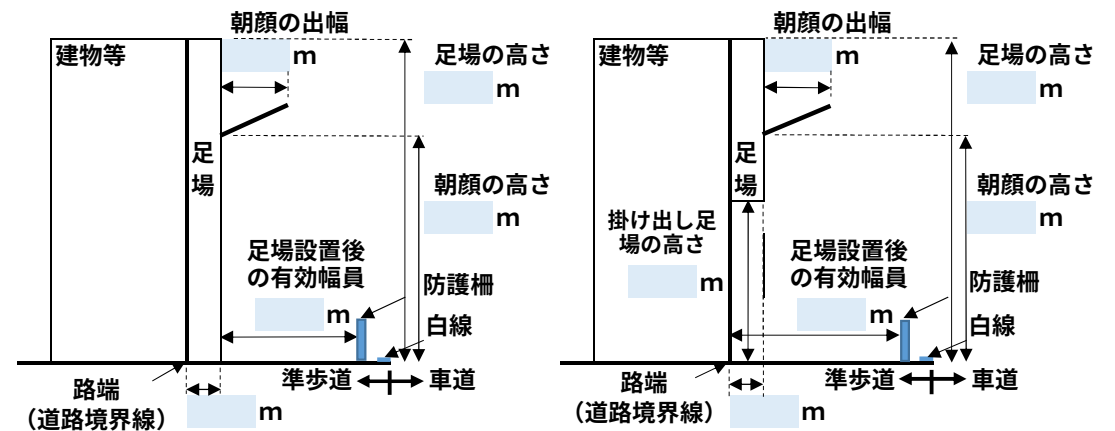
断面図 (側面図)
