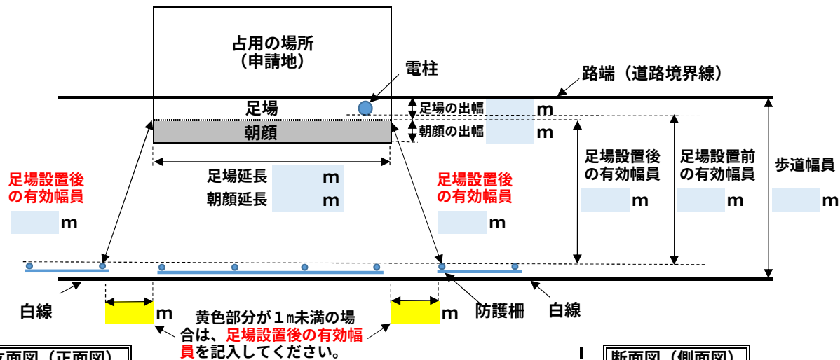
立面図 (正面図)
