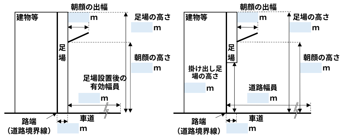
断面図 (側面図)
