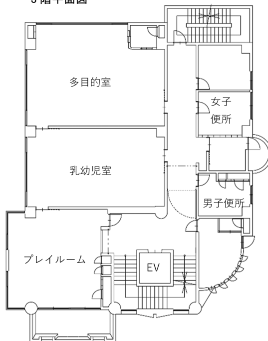
3 階平面図
