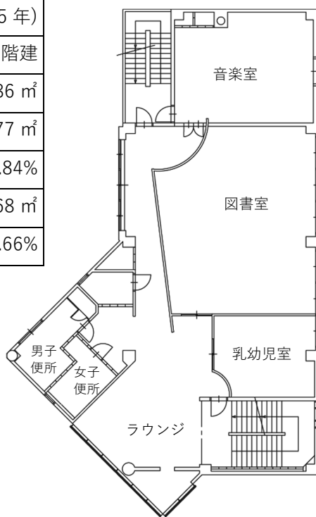
2 階平面図
