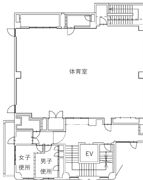
4 階平面図
