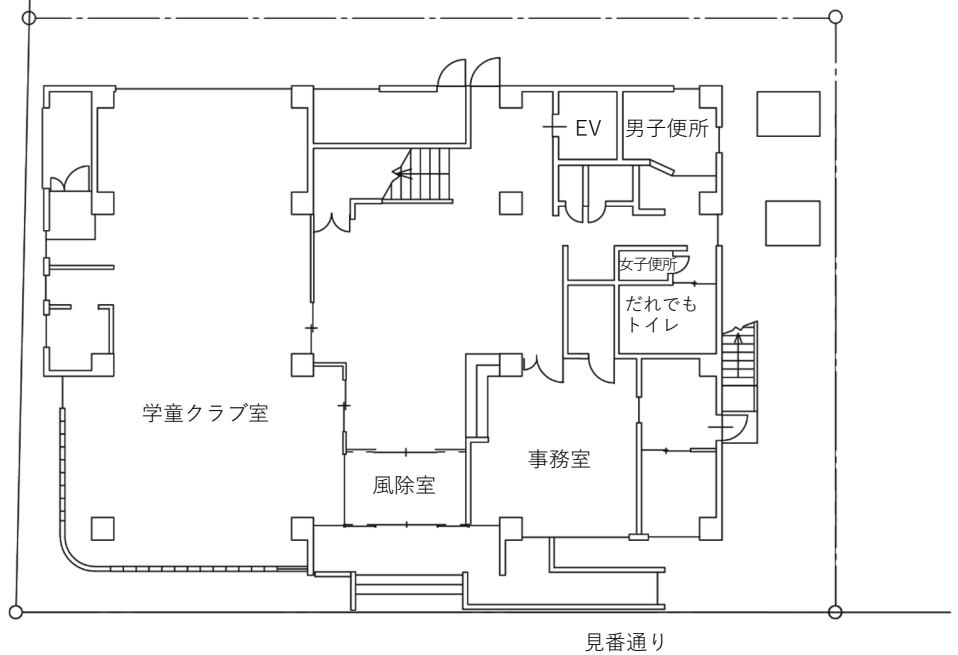
1 階平面図
