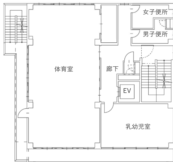
4 階平面図
