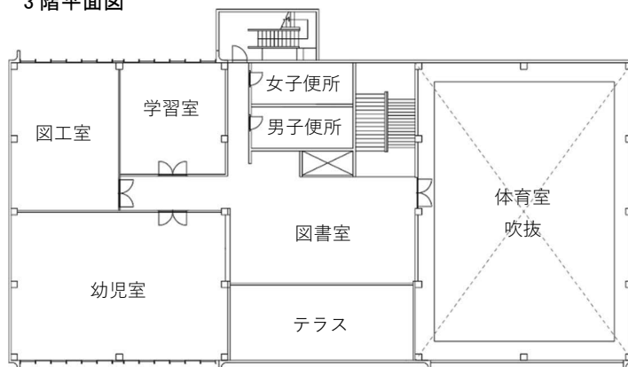
3 階平面図
