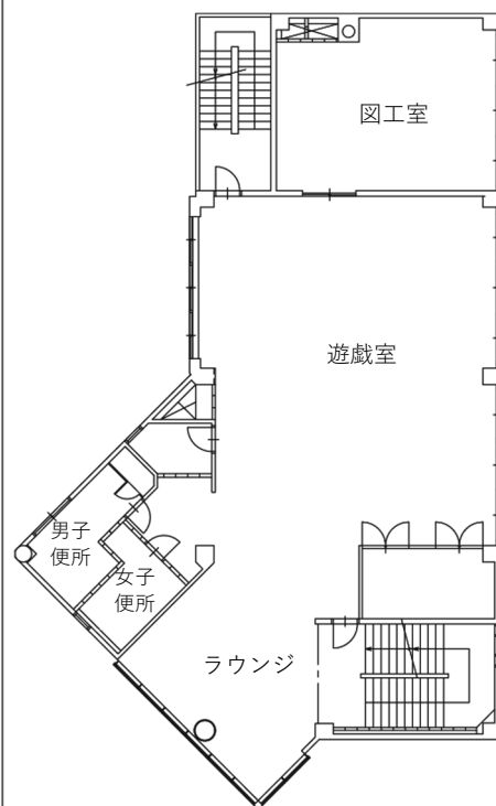
3 階平面図
