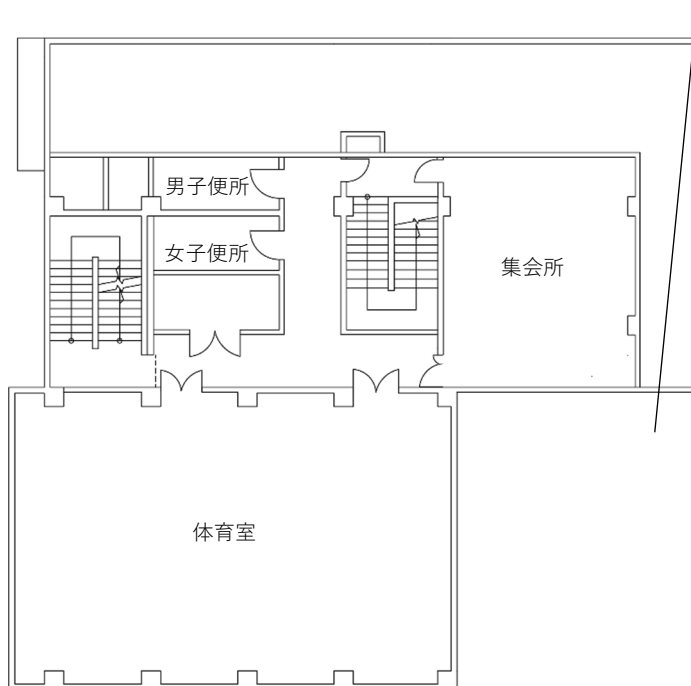
3 階平面図
