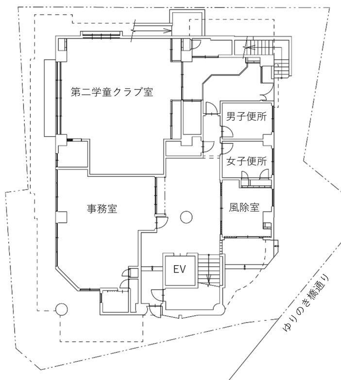
2 階平面図
