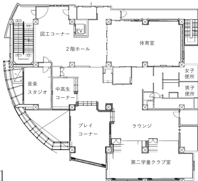
2 階平面図
