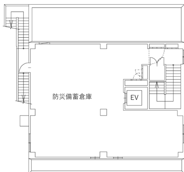
4 階平面図
