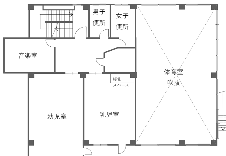
3 階平面図
